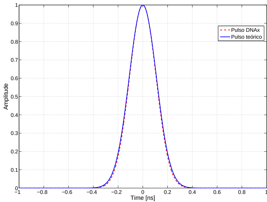
Figura 5.16: Pulso UWB singelo gerado pela técnica DNax.
