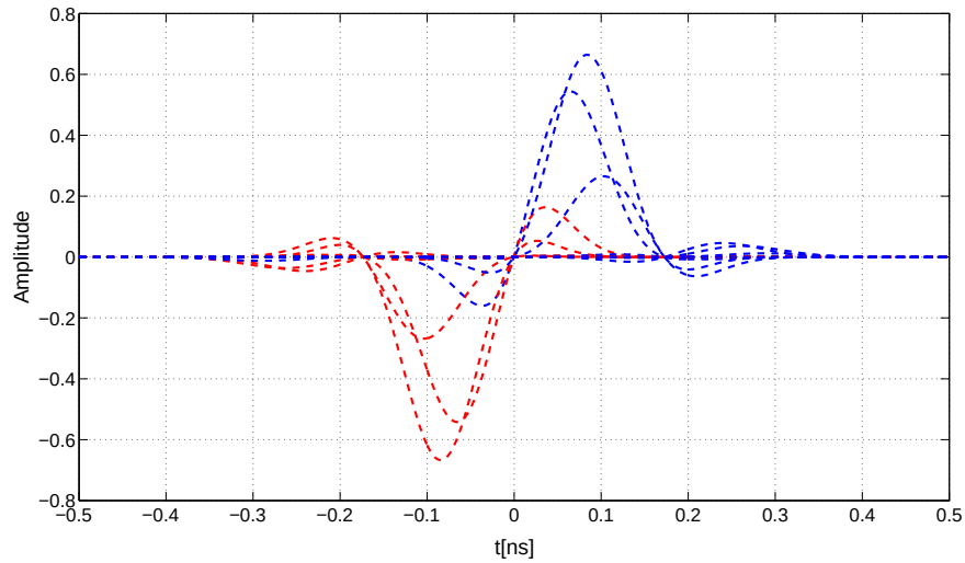
Figura 5.3: As formas de ondas geradas pela técnica DNax ponderadas pelo coeficiente C_k e deslocadas de kd .
