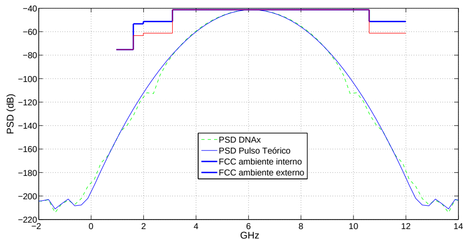
Figura 5.17: Densidade espectral de potência do pulso singelo.
