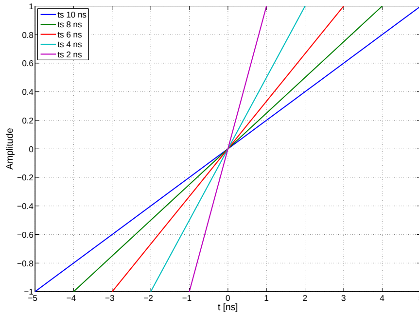
Figura 5.15: Exemplos da função base geradora x(t) .
