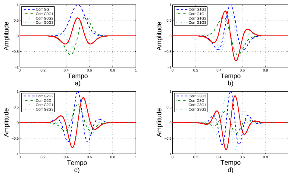
Figura 4.6: Resultado da correlação entre os pulsos Gaussiano, Monociclo, Doublet e a 3ª derivada do pulso Gaussiano.
